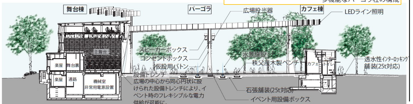
公園全体断面図 No-Scale
