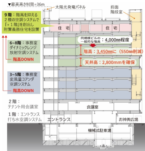
上) 変風量コアンダ空調システム…壁面上部より空気を送り出す。天井は空気を這わせるため、平滑な仕上げになっている。 右) 断面ダイアグラム。「+1フロア」で付置義務である住宅階を創出し、必要なオフィス面積を確保。
