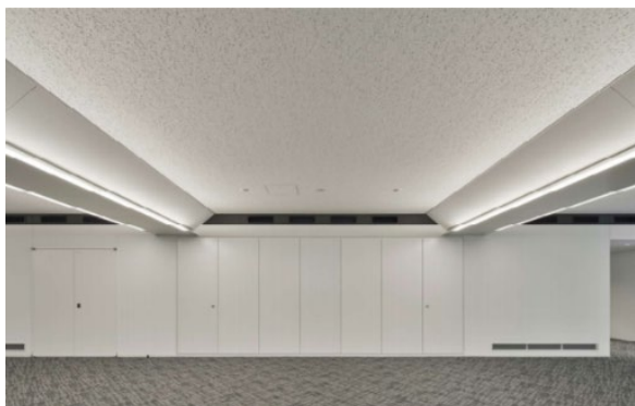
上) 変風量コアンダ空調システム…壁面上部より空気を送り出す。天井は空気を這わせるため、平滑な仕上げになっている。 右) 断面ダイアグラム。「+1フロア」で付置義務である住宅階を創出し、必要なオフィス面積を確保。
